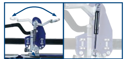
Piston à gaz pour une pression parfaite
