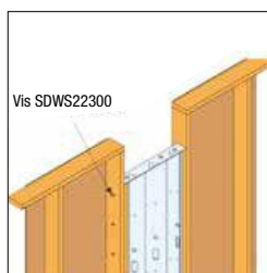
Etape 3 Liaison avec les montants adjacents
