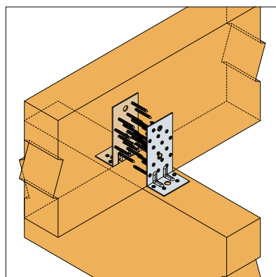
Fixation bois/bois type poutre/poutre
