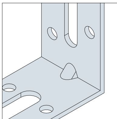
Équerre de fixation avec raidisseur
