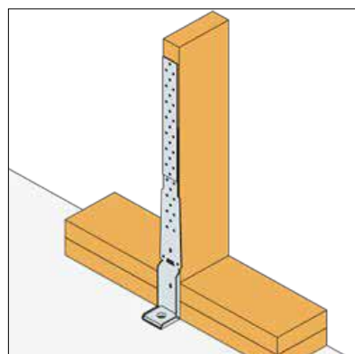
Clouage minimum - configuration pliée
