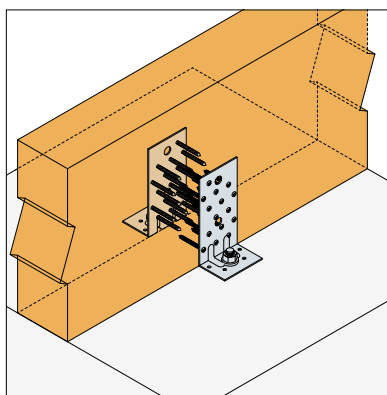
Fixation bois/support rigide type poutre
