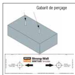
Etape 1 Mise en place des tiges filetées
