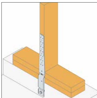
Clouage minimum - configuration à plat
