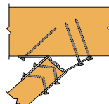
3 - Clouage sur l'élément porteur
