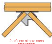
2 arêtiers simple sans empañon
